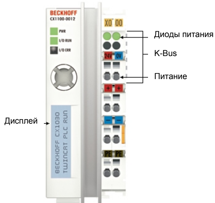
Блок питания с K-bus интерфейсом
