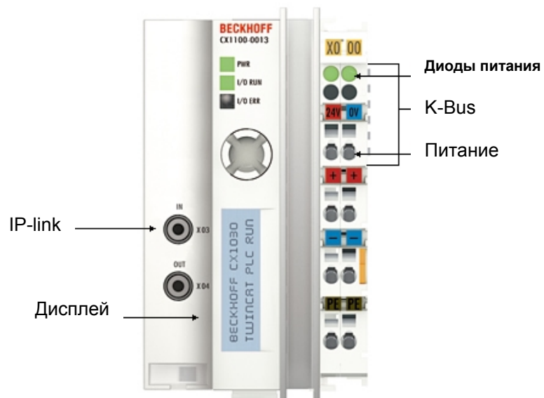
Блок питания с K-bus и IP-Link интерфейсами
